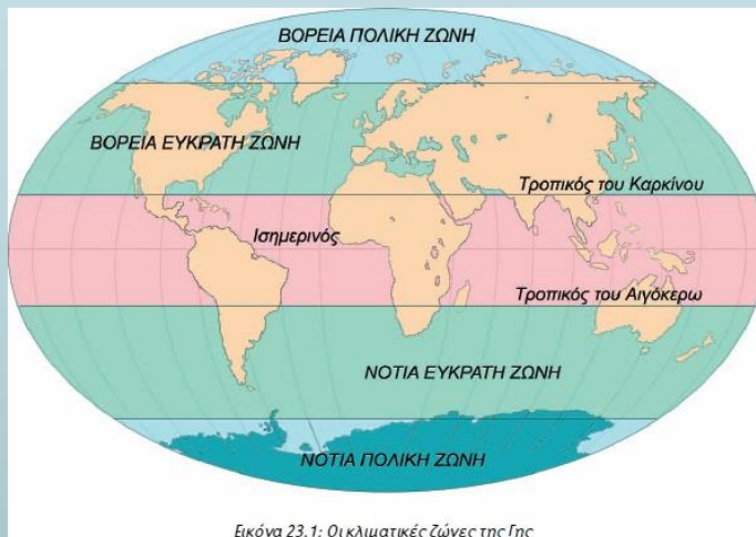
Εικόνα 23.1: Οι κλιματικές ζώνες της Γης
